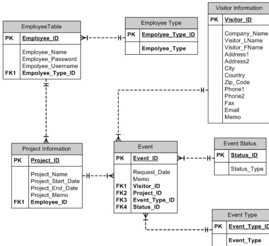
รูปตัวอย่างของ E-R Diagram
