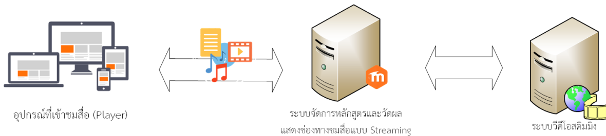
รูปแสดงการทำงาน Streaming ของโครงการ
