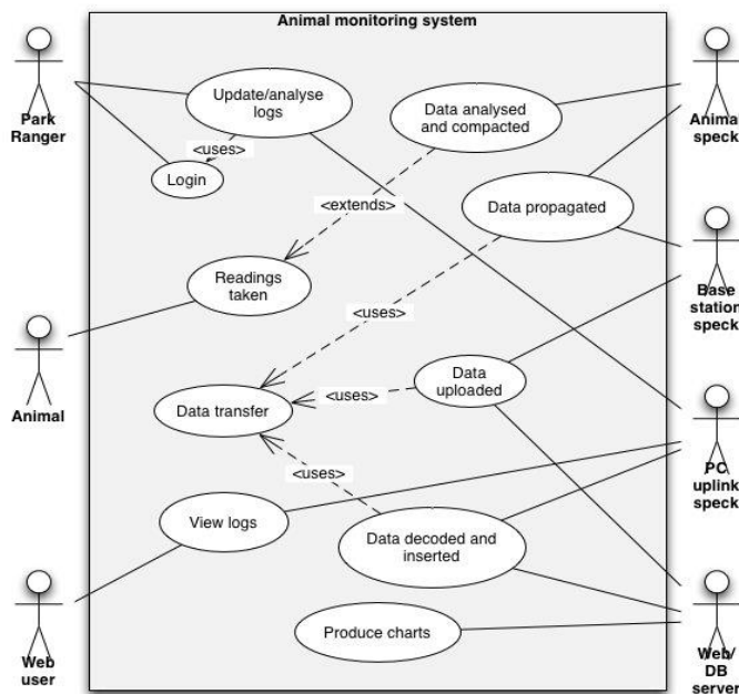
ภาพที่ 1 รูปตัวอย่างของ Use case
