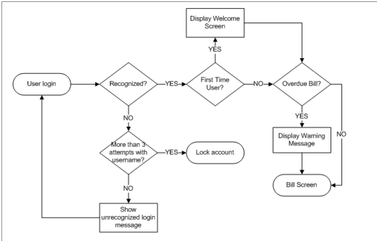
รูปตัวอย่างของ Work flow
