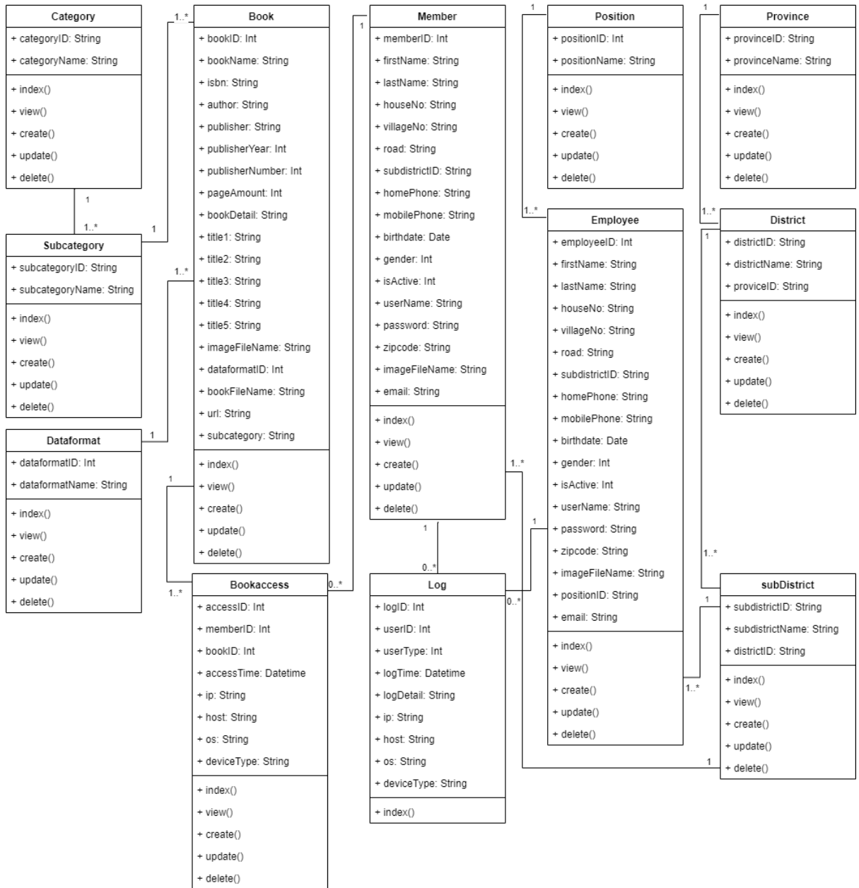
ภาพที่ 3.3 คลาสไดอะแกรม
