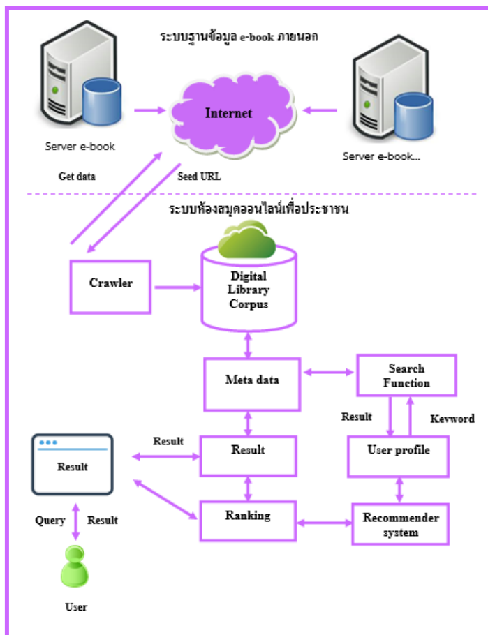
ภาพที่ 3.21 สถาปัตยกรรมการพัฒนาการพัฒนาระบบการแนะนำหนังสือของระบบห้องสมุดออนไลน์
