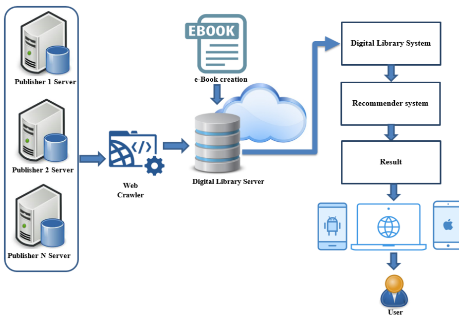
ภาพที่ 3.20 แสดงกระบวนการทำงานของระบบห้องสมุดออนไลน์
