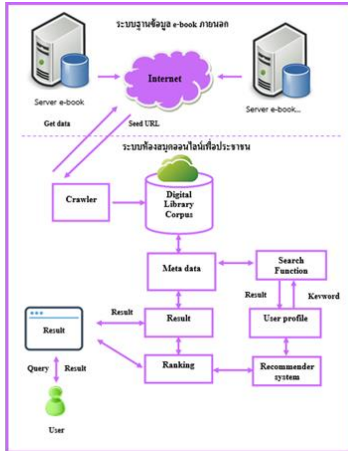
ภาพที่ 6 สถาปัตยกรรมการพัฒนากระบวนการแนะนำหนังสือของระบบห้องสมุดออนไลน์
