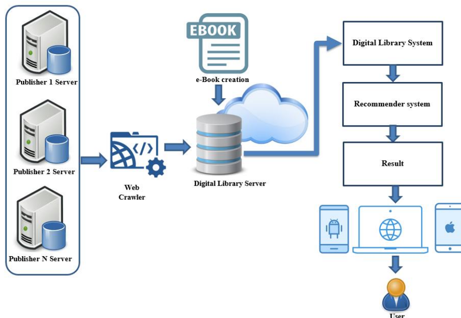
รูปที่ 4 กระบวนการทำงานระบบห้องสมุดออนไลน์
