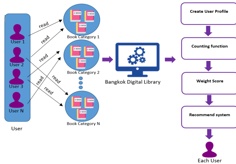
ภาพที่ 8 กระบวนการแนะนำหนังสือให้กับผู้ใช้แต่ละคน
