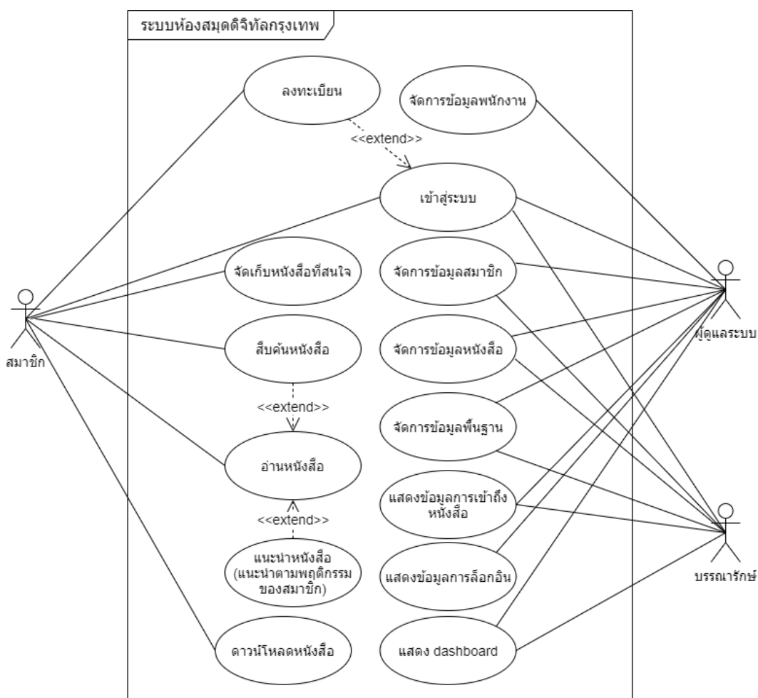
ภาพที่ 3.2 ยูสเคสไดอะแกรม
