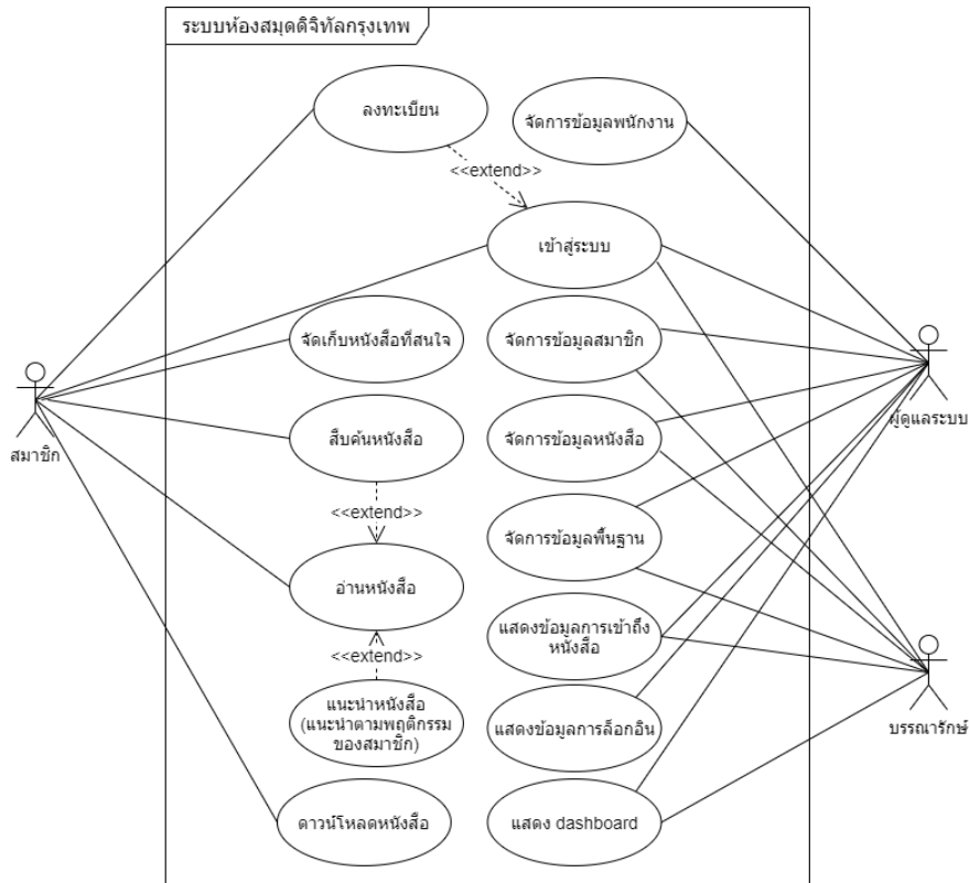
ภาพที่ 3 ยูสเคสไดอะแกรม
