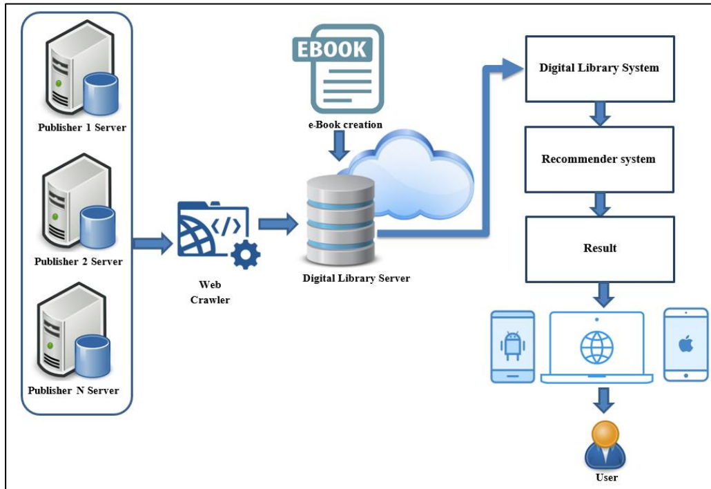
รูปที่ 21 แสดงกระบวนการการเชื่อมโยงระบบกับฐานข้อมูลอื่นๆ
