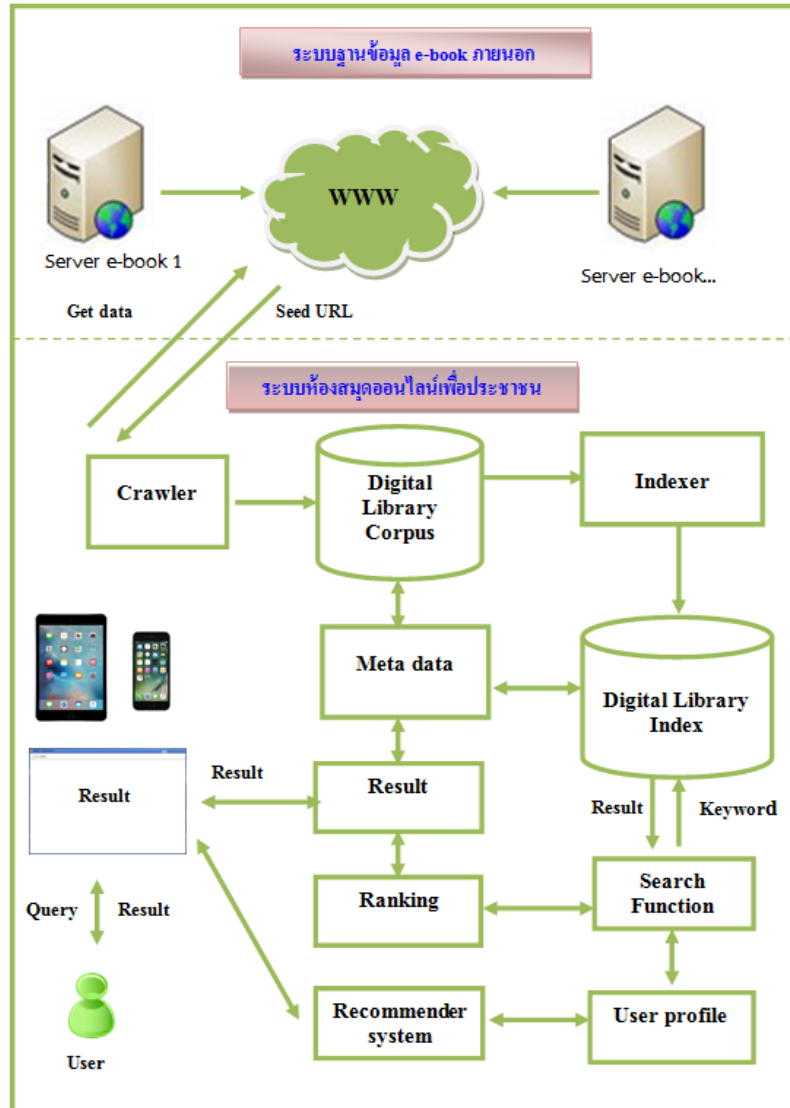
รูปที่ 6 สถาปัตยกรรมการพัฒนาห้องสมุดออนไลน์
