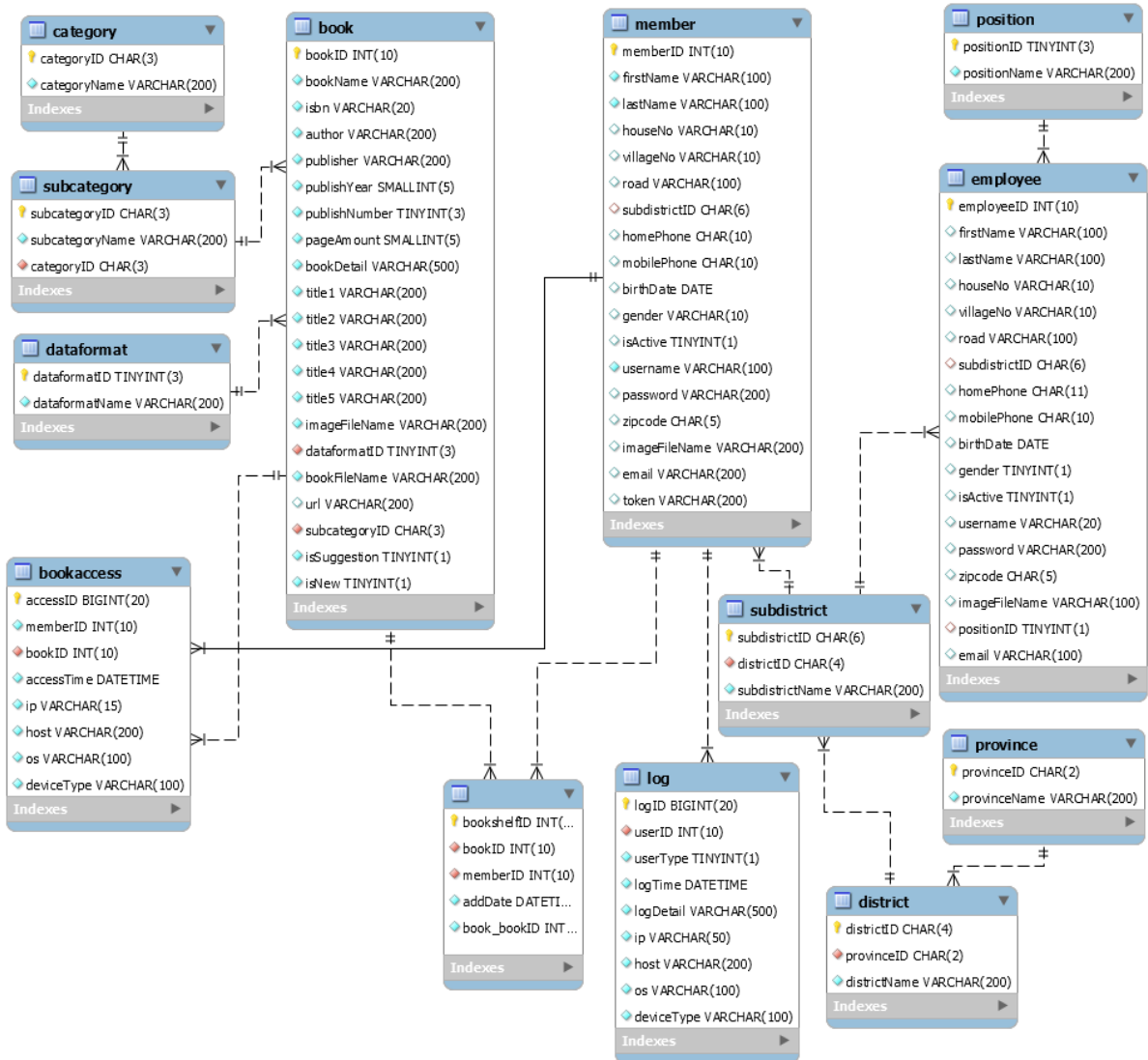
รูปที่ 3 แผนภาพความสัมพันธ์ระหว่างเอนทิตี
