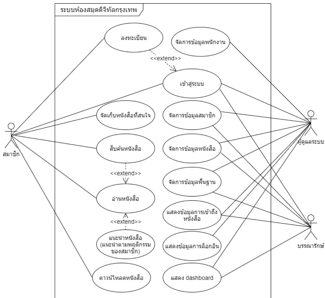
รูปที่ 1 ยูสเคสไดอะแกรม
