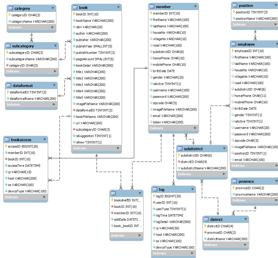
ภาพที่ 4 แผนภาพความสัมพันธ์ระหว่างเอ็นทิตี
