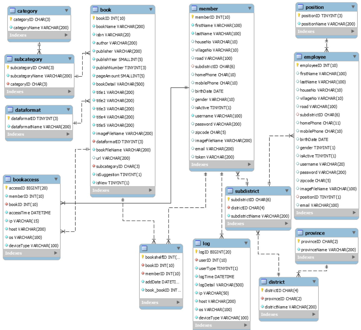
ภาพที่ 3.4 แผนภาพความสัมพันธ์ระหว่างเอนทิตี
