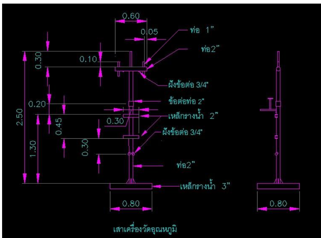
ภาพที่ 89 แสดงภาพโครงร่างวิศวกรรมของเสาสำหรับติดตั้งสถานี
