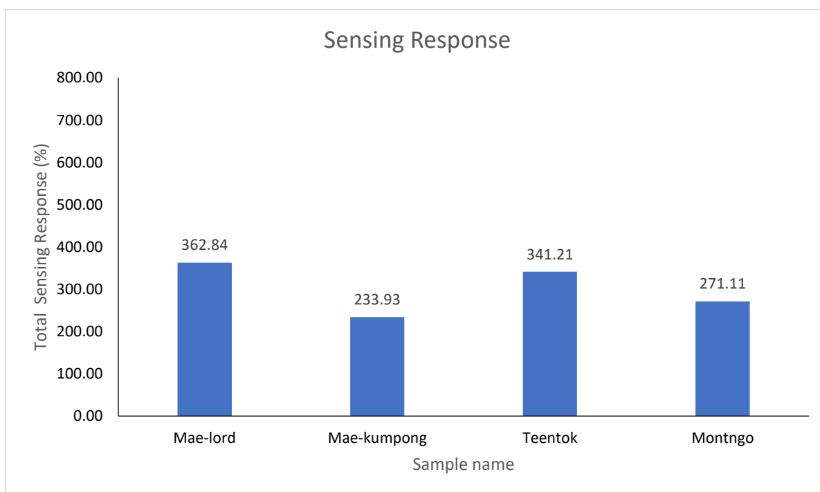
ภาพที่ 170 แสดงอัตราการตอบสนองรวมของก๊าซเซนเซอร์ต่อกลิ้นเมลิ็ดกาแฟคั่ว
