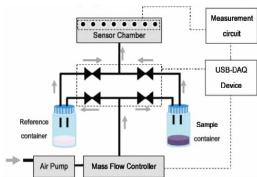
ภาพแสดงองค์ประกอบของเครื่องจมูกอิเล็กทรอนิกส์ (Electronic Nose)
